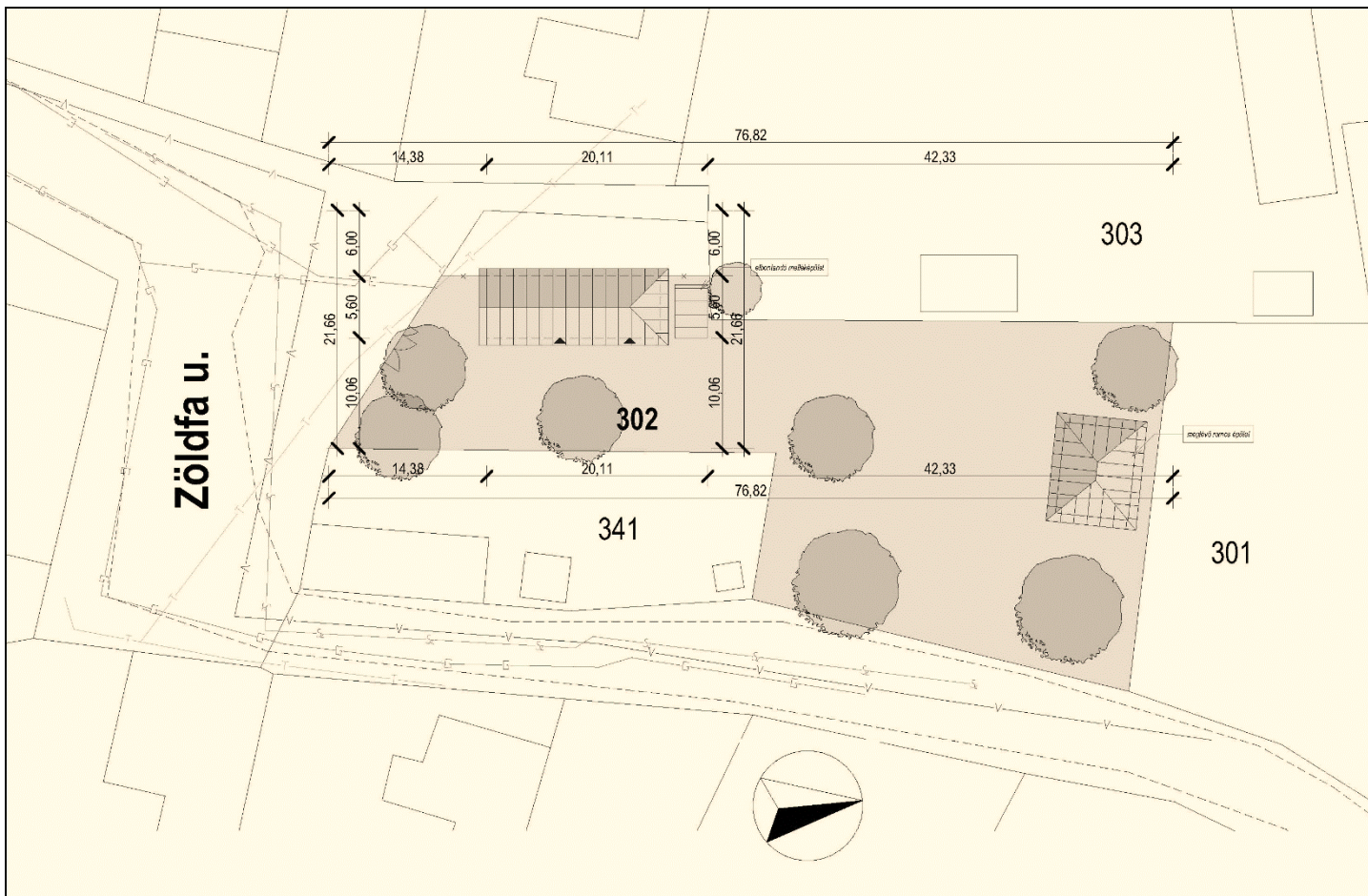
1. ábra. Helyszínrajz (A felmérést készítette: Sáth Péter, 2026.)
