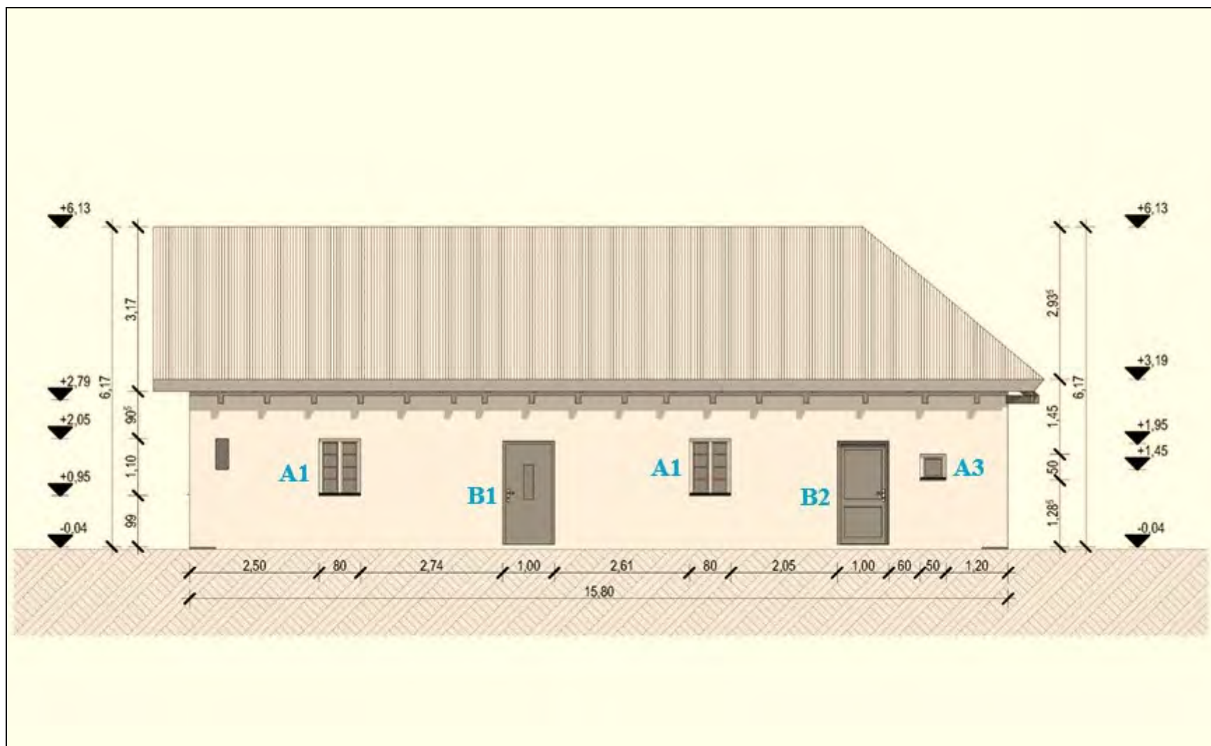
3. ábra. Keleti (udvari) homlokzat (A felmérést készítette: SÁTH Péter, 2026.)
