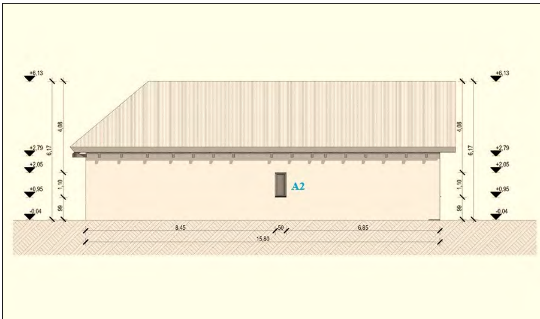
4. ábra. Nyugati homlokzat (A felmérést készítette: SÁTH Péter, 2026.)
