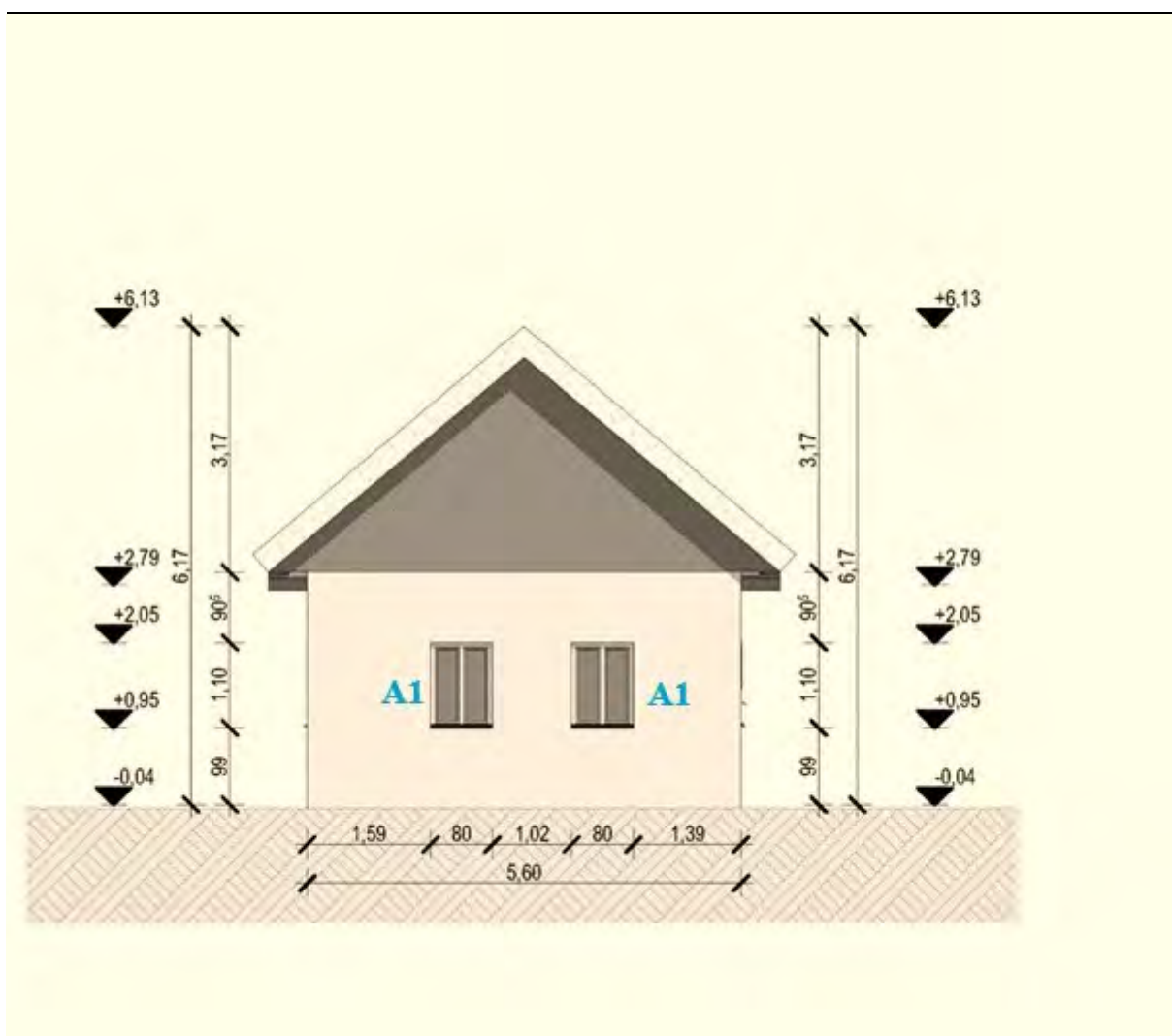
5. ábra. Déli homlokzat (A felmérést készítette: Sáth Péter, 2026.)
