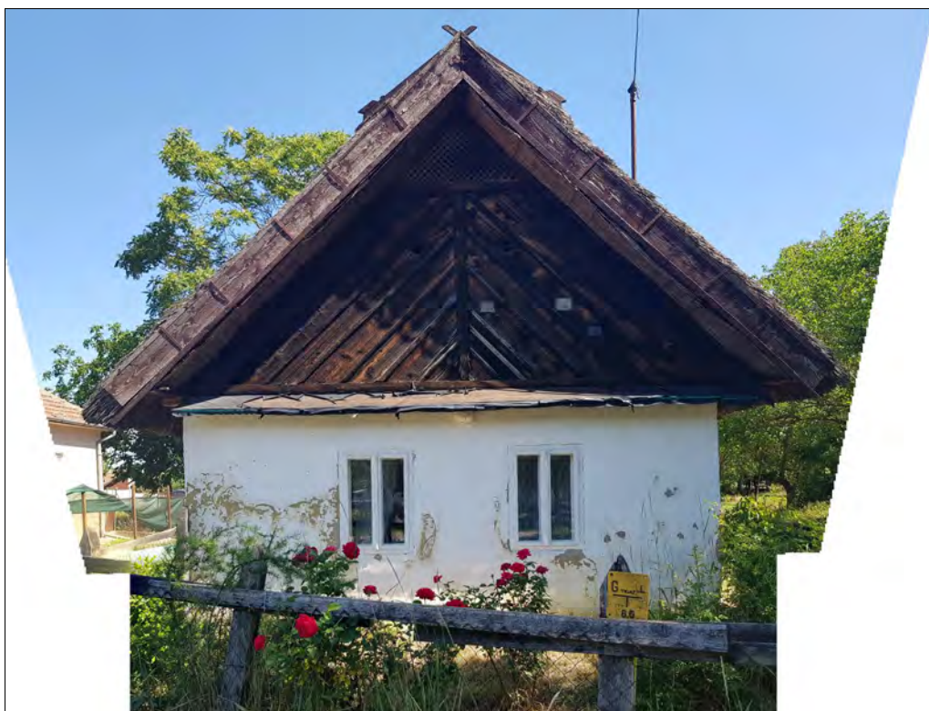
12. kép. A népi lakóépület déli homlokzata
